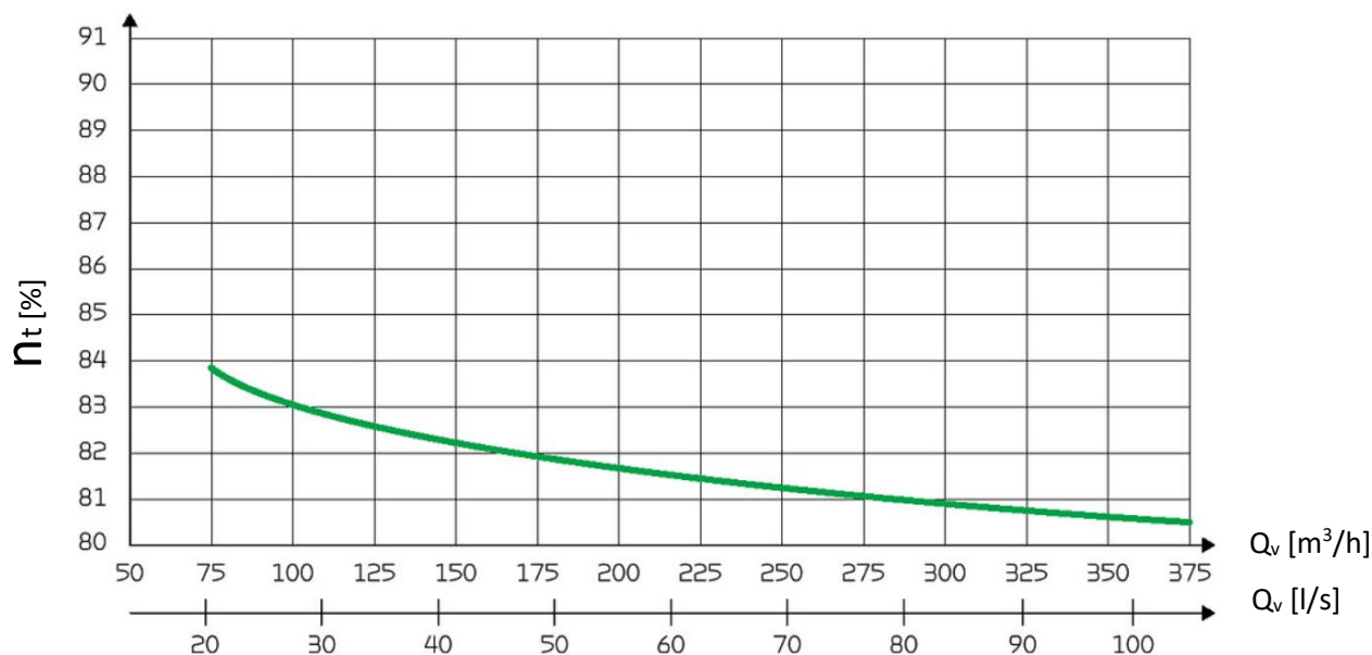
Účinnost (EN 308)
