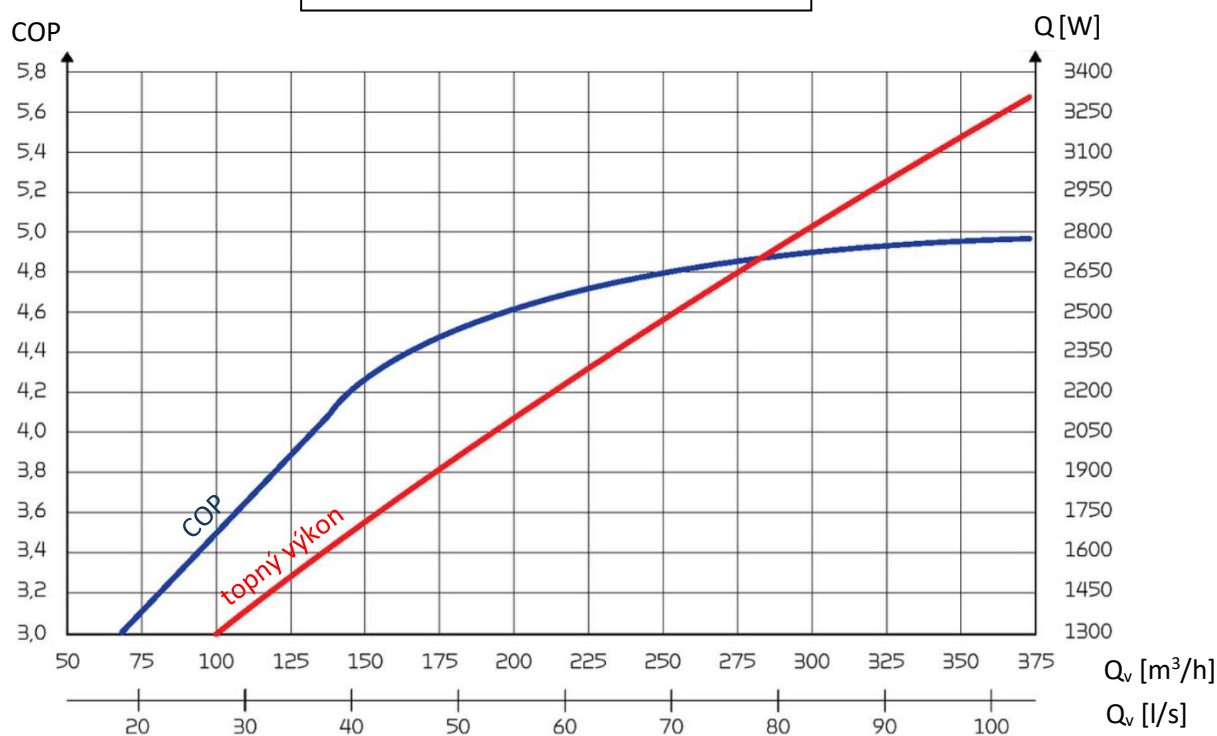
COP (EN14511), odtah 21 °C
